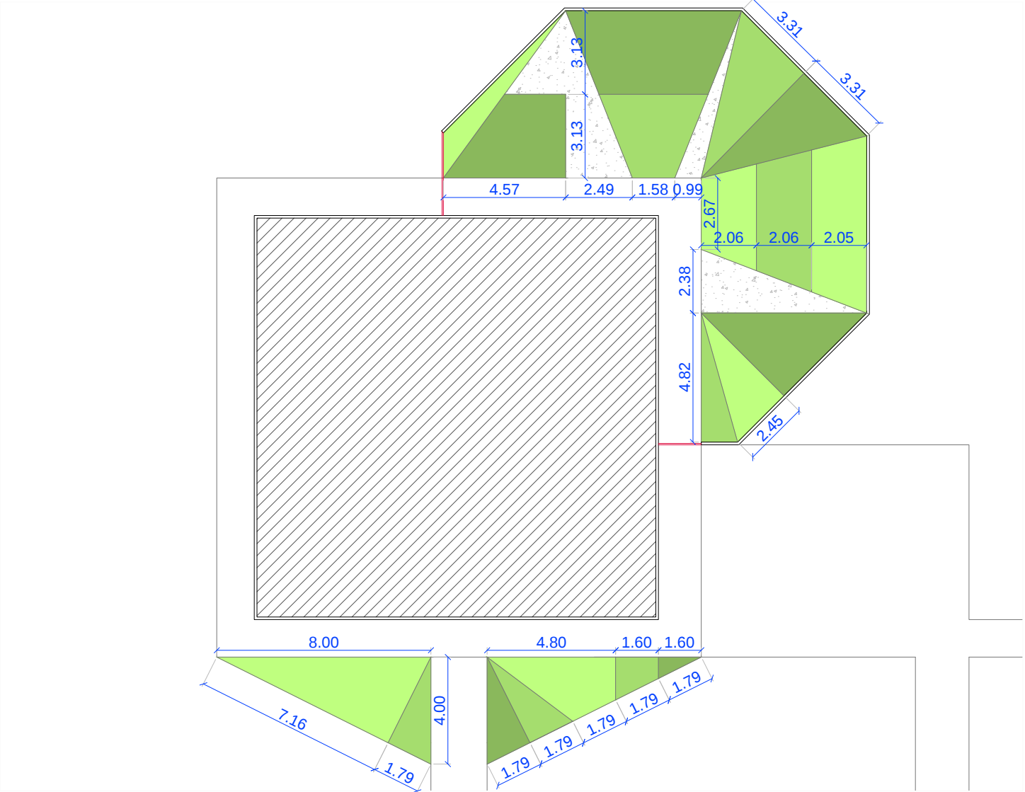
Planta de Vegetação Escala: 1.200
