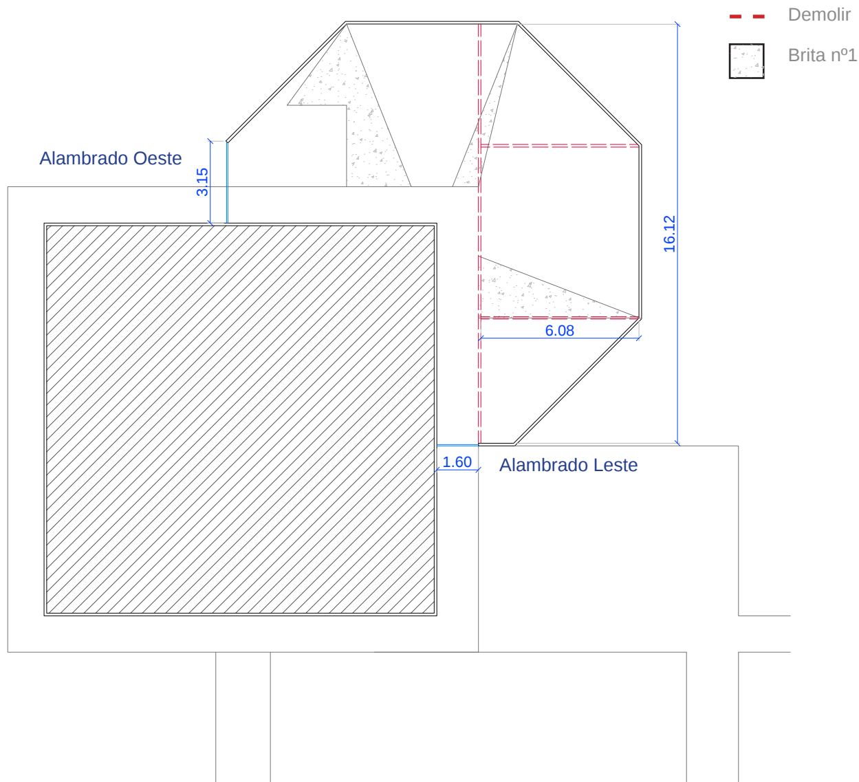
Planta Construir/Demolir Escala: 1.200
