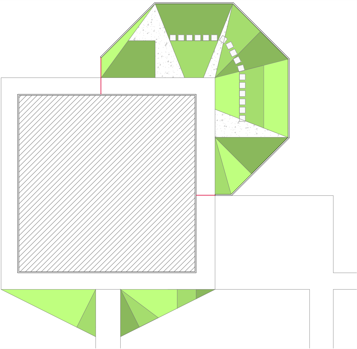
Planta de Vegetação Escala: 1.200
