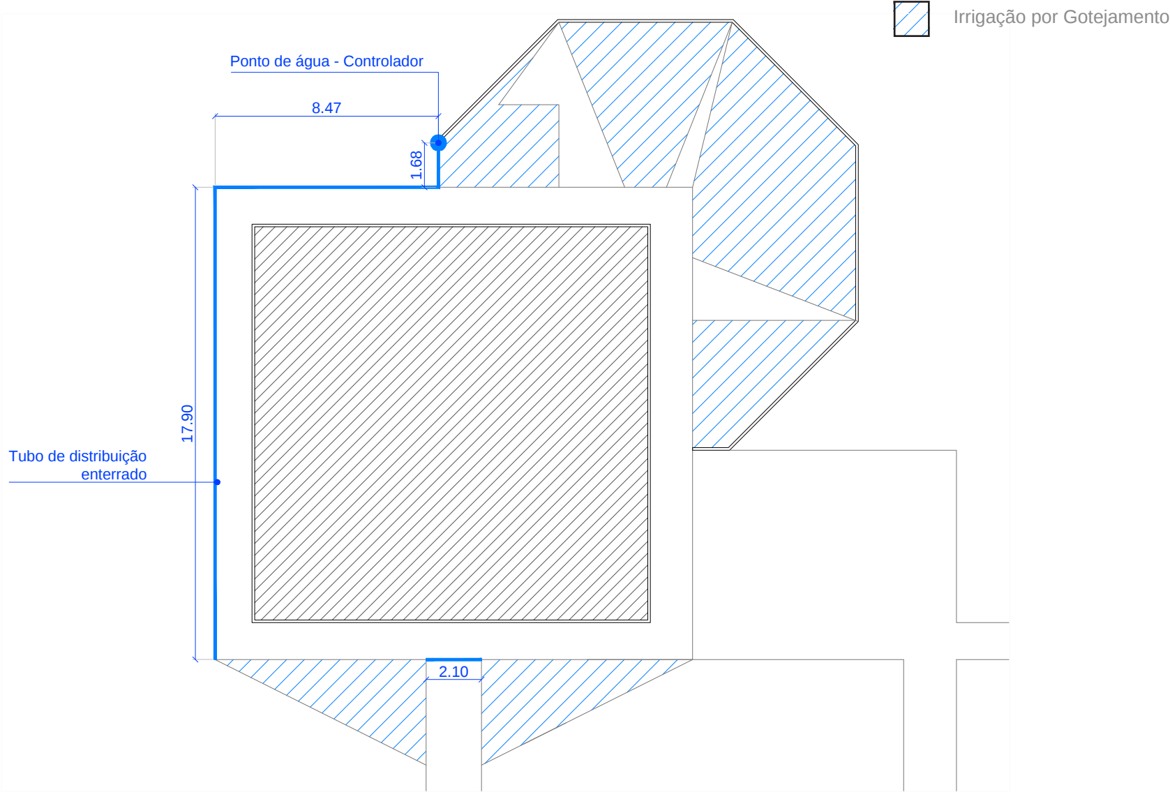
Planta de Irrigação Escala: 1.200
